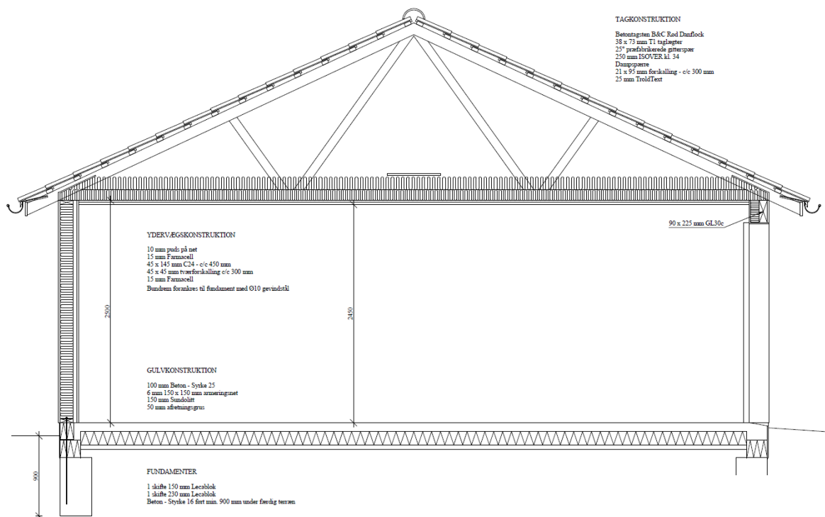
Figur 4. Garage snit tegning
